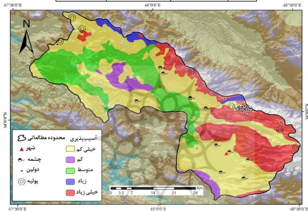
شکل ۹. پهنه‌بندی نهایی آسیب‌پذیری آبخوان‌های محدوده تاقدیس گرین به روش PaPRIKa
