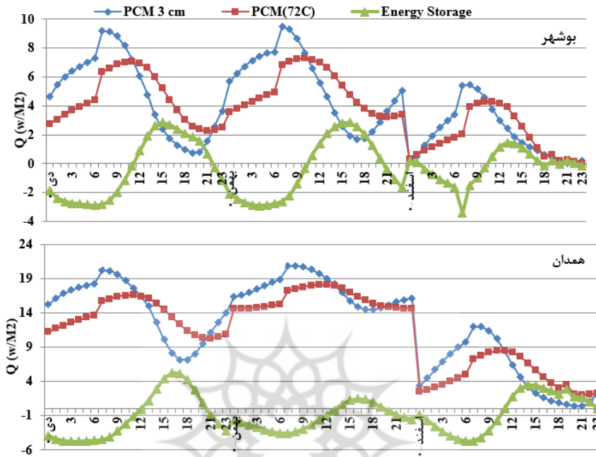
شکل ۱۰. مقایسه‌ی شار حرارتی آبی اقلافی در زمستان در بوشهر و همدان
