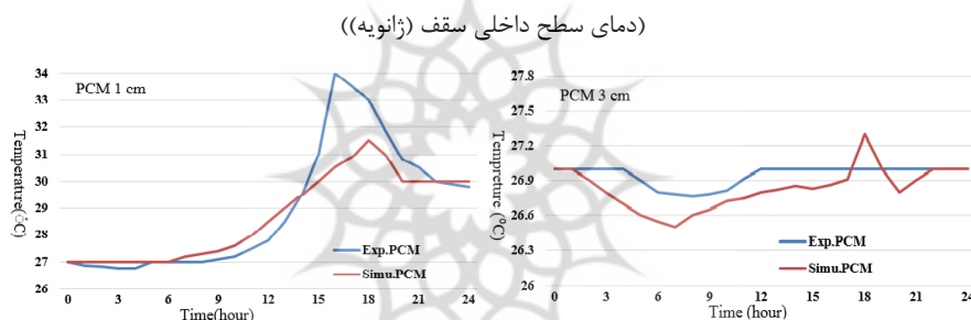
شکل ۵. مقایسه‌ی نتایج تجربی (پسوپاتی، ۲۰۰۸) و شبیه‌سازی سقف اتاق با ماده تغییر فاز دهنده
