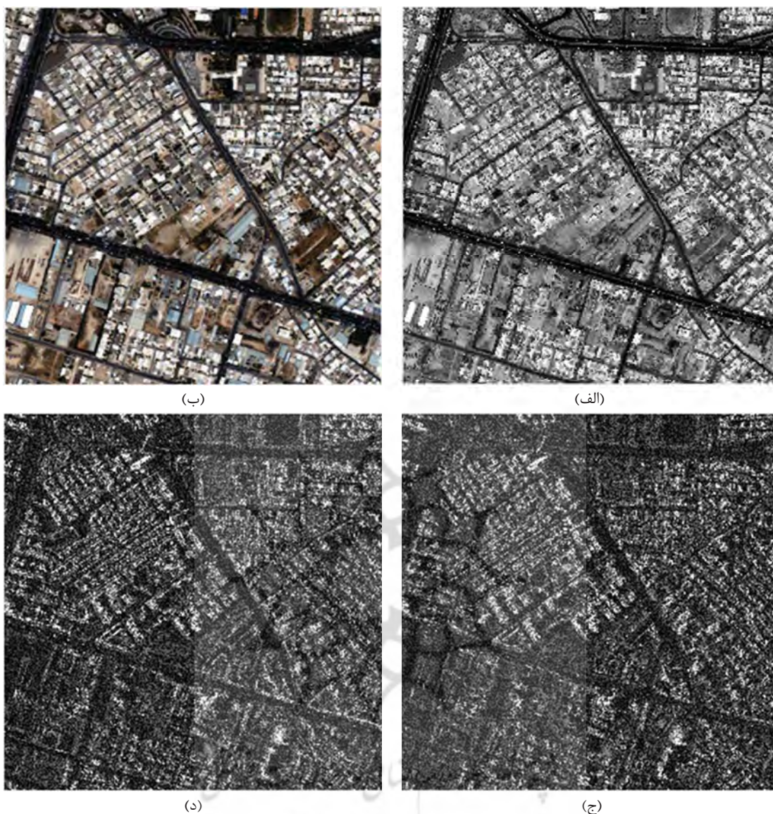
شکل ۳. تصاویر منطقه دوم: تصویر پانکروماتیک ماهواره آیکنونوس (الف)؛ تصویر چندطیفی ماهواره آیکنونوس (ب)؛ تصویر SAR در پلاریزاسیون HH (ج)؛ تصویر SAR در پلاریزاسیون VV (د)
