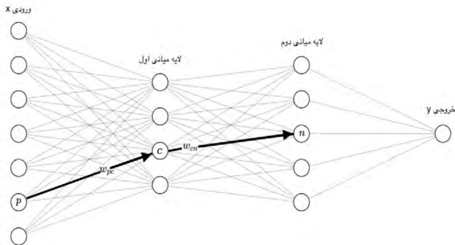
شکل ۲- ساختار شبکه عصبی با ۲ لایه پنهان
