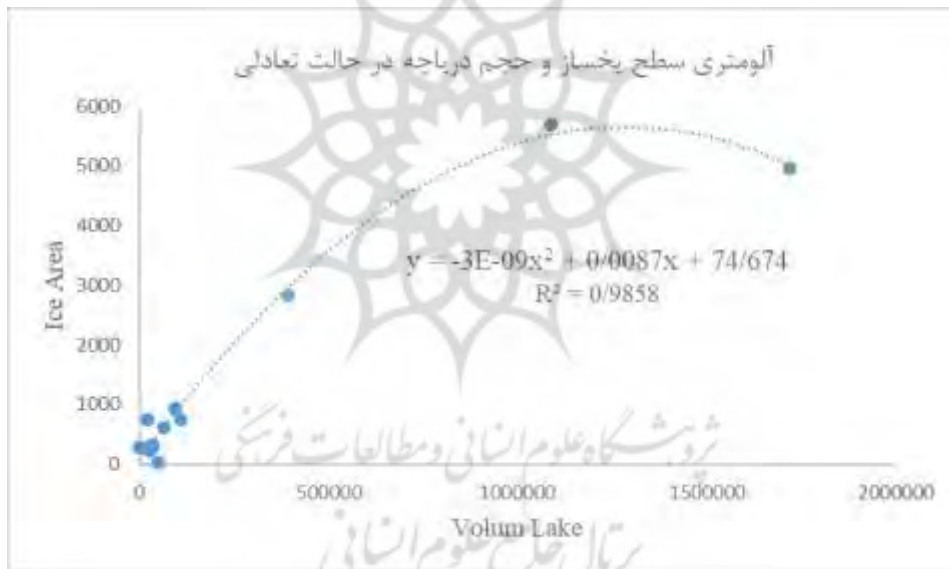
شکل ۳- گراف آلومتری توانش محیطی (حجم دریاچه و سطح یخساز)
