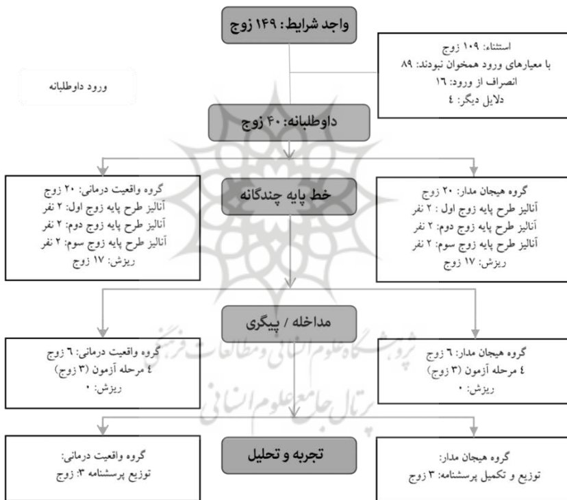
نمودار ۱. نمودار جریان فرآیند نمونه‌های آماری
