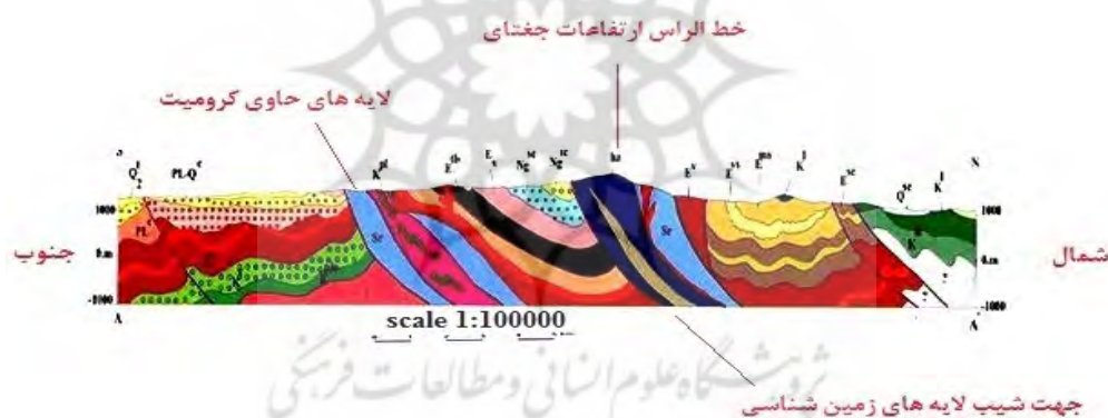
شکل (۶). نیمرخ زمین شناسی از ارتفاعات جغتای. (منبع: نگارندگان، ۱۳۹۷)
