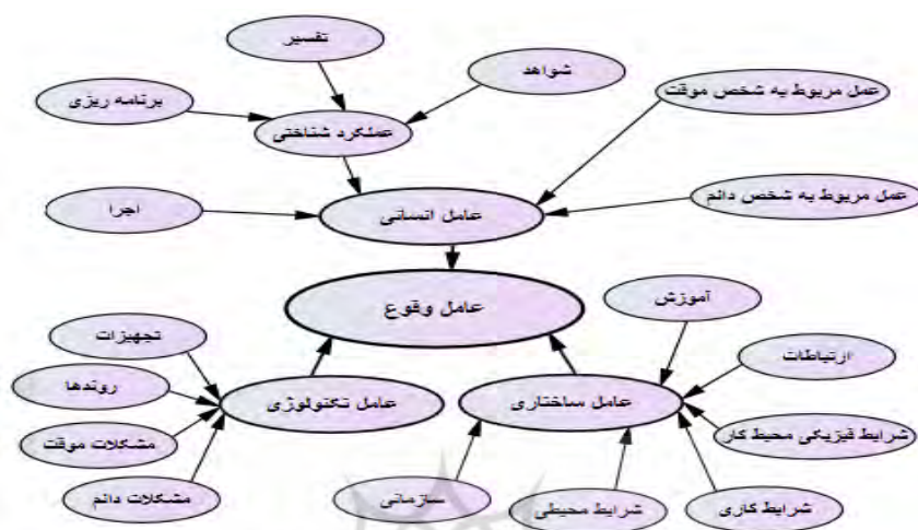
شکل ۱. ساختار نظری تحقیق و چگونگی استفاده از آن برای اندازه‌گیری احتمال وقوع یا شدت وقوع یک حادثه، از دیدگاه خیرگان
