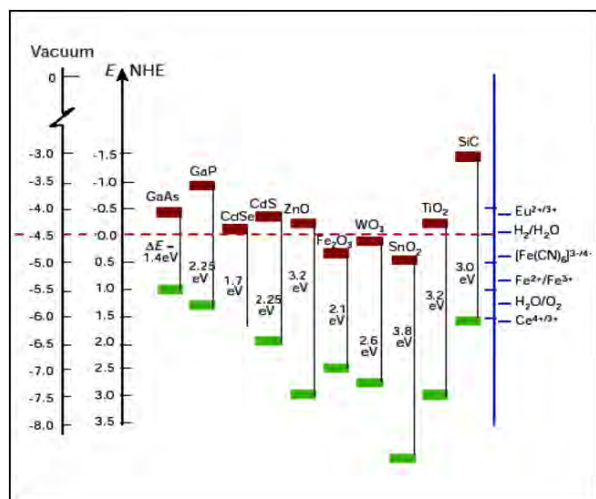
شکل ۳- سطوح انرژی نوار ظرفیت و نوار هدایت چند نیمه‌هادی در محلول آبی با \text{pH} = 1 .
