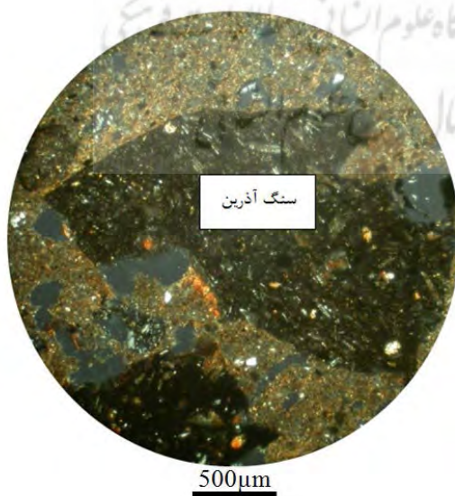
تصویر ۸. تصویر میکروسکوپی نمونه شماره ۷ کورا-ارس، نور XPL، طول میدان دید 2.7mm، بافت پورفیری، انواع مختلف قطعات درشت سنگ‌های آذرین بیرونی در زمینه سفال (نگارندگان، ۱۳۹۹).
