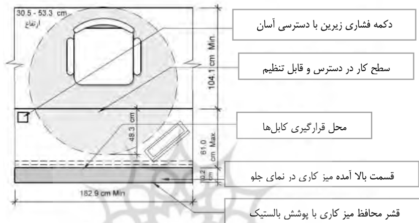
شکل ۱ طرح پلان جایگاه نشستن قاضی (منبع: نشریه ۷۸۱ ص ۸۹)
