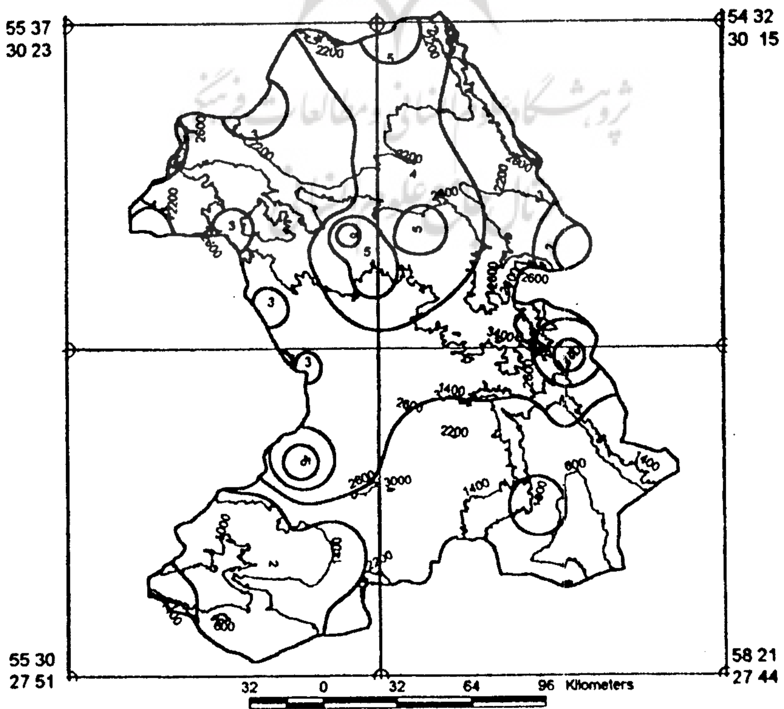
شکل ۵- نقشه همبارش دو روزه در منطقه
