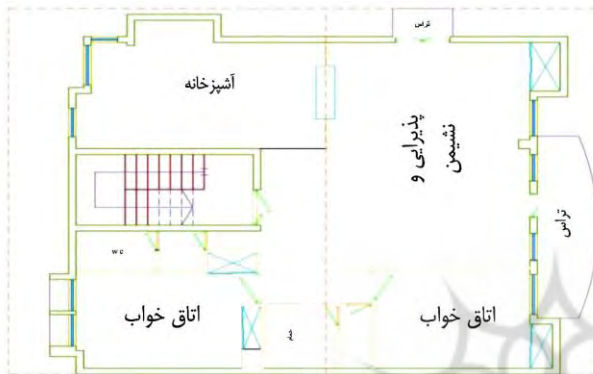
تصویر ۹- پلان طبقه سوم و نیمه طبقه بالای طبقه سوم خانه‌ای در کوچه مختاران
