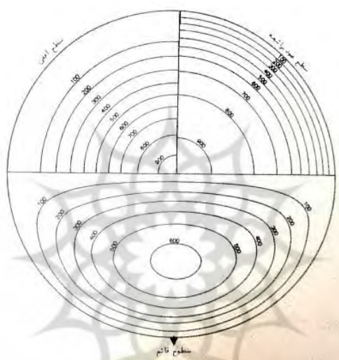
تصویر ۱- نقاله انرژی خورشیدی (قیابکلو، ۱۳۹۴)
