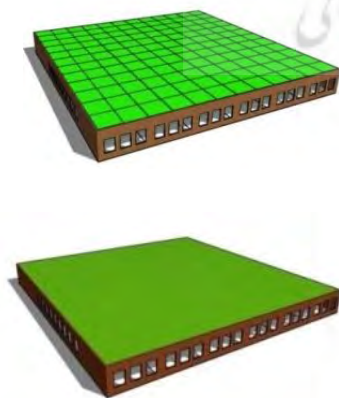
تصویر ۵- شبیه‌سازی هندسی پیرامون سنجش تفاوت دو نمونه بام سبز هیدروپونیک گسترده و مدولار از نظر صرفه‌جویی در مصرف انرژی حرارتی مدارس در مدارس سبز اقلیم سرد و خشک ایران
