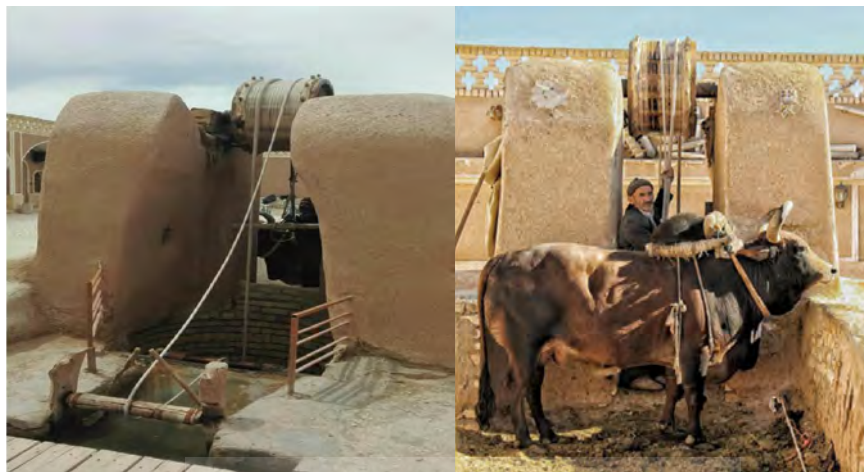
عکس ۵- بدنی اصلی چاه (کاکوچاه) در گاوجاه حاج ابراهیم (ورزنه)
