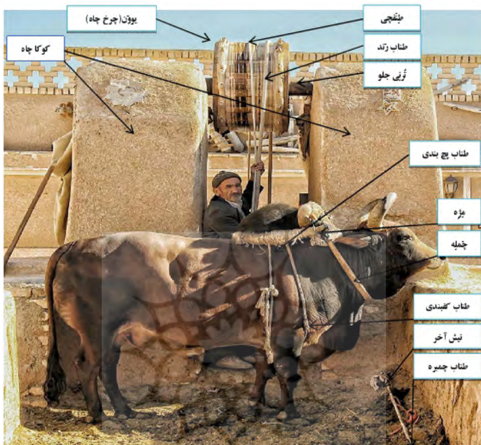
عکس ۶- اجزا و عناصر تشکیل دهنده بدنی اصلی چاه (کاکوچاه) در گاوچاه حاج ابراهیم
