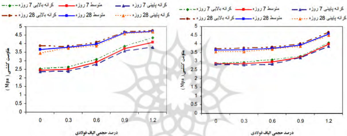
شکل ۶- سمت راست: مقاومت کششی ۷ و ۲۸ روزه نمونه استوانه ای ۱۵۰×۷۵×۷۵ mm و سمت چپ: مقاومت کششی ۷ و ۲۸ روزه نمونه منشوری شکل ۱۰۰×۱۰۰×۵۰ mm (وظیفه خواه و مناف پور، ۱۳۸۹)
