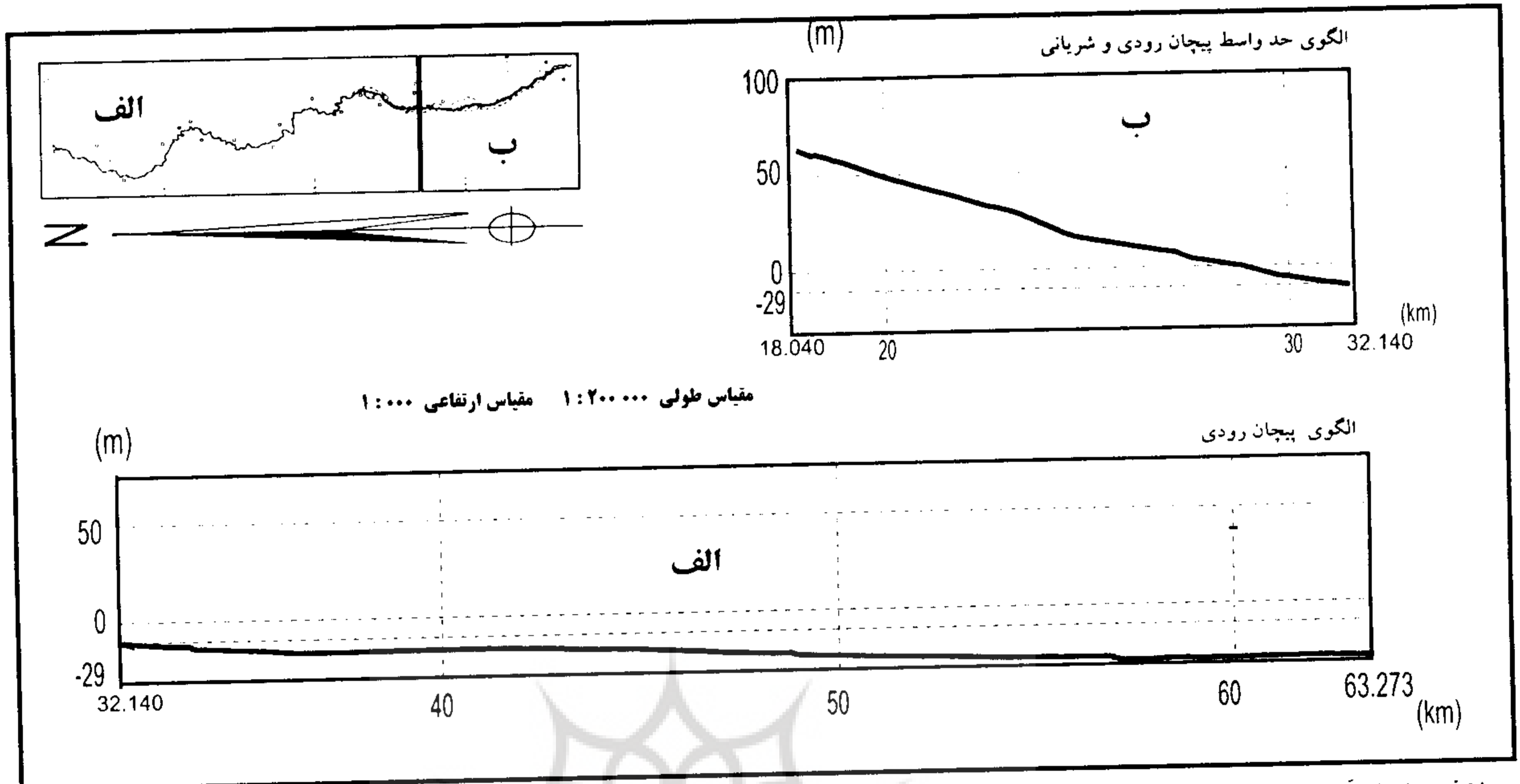
شکل ۱- نیمرخ طولی رودخانه تالار
