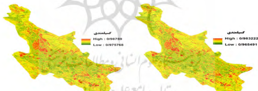
شکل (۹): گسیلمندی حساب شده برای داده زمستان، سمت راست برای بانده ۱۳ و سمت چپ برای بانده ۱۴
