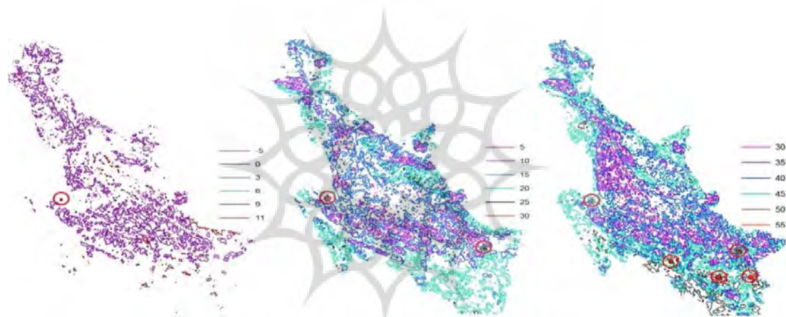
شکل (۲۰): نقشه خطوط همدمای منطقه مورد مطالعه، از سمت راست تصویر تابستان روز، زمستان روز و زمستان شب
