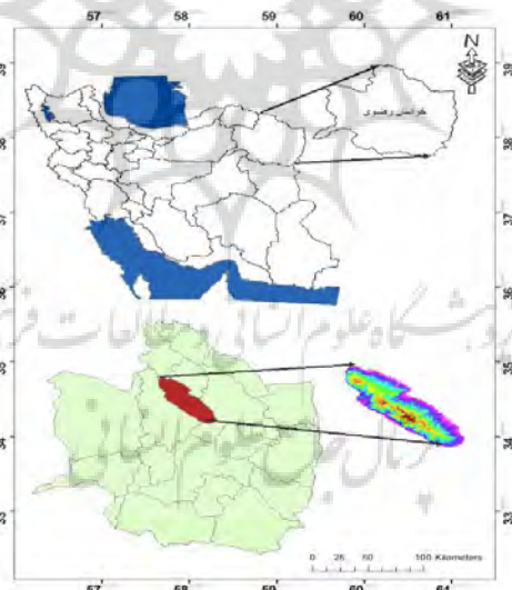
شکل (۱): موقعیت منطقه مورد مطالعه
