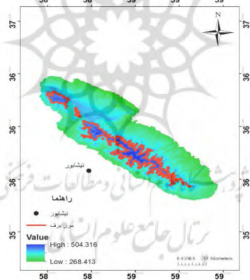
شکل (۷): نقشه تفاوت دمایی بین زمان حاضر و دوره پلیستوسن در محدوده مورد مطالعه
