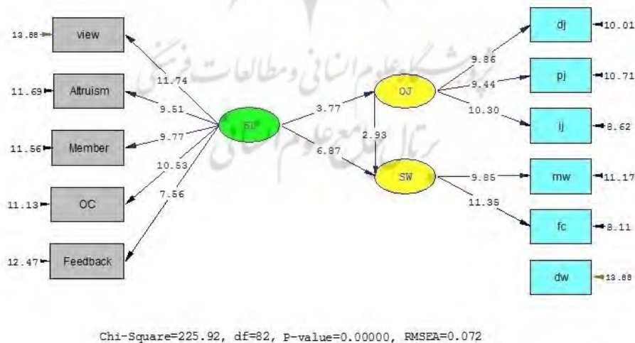
شکل ۲: مدل معادلات ساختاری در حالت اعداد معناداری
