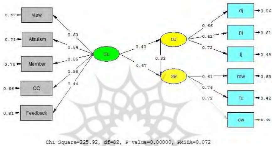
شکل ۱: مدل معادلات ساختاری در حالت استاندارد
