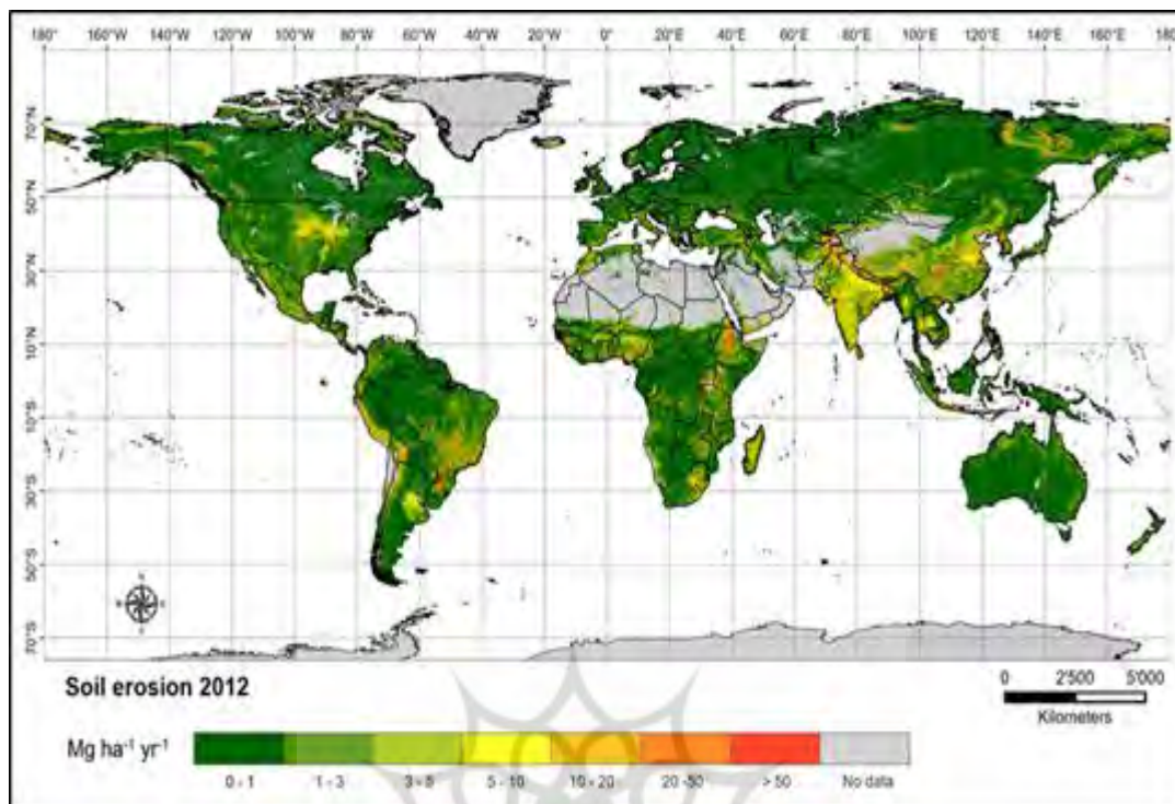
نقشه ۲: روند فرسایش خاک در جهان
