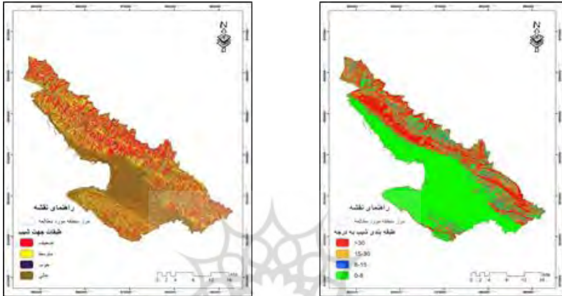
شکل ۱۸- طبقه بندی شیب محدوده مورد مطالعه شکل ۱۹- طبقات جهت شیب محدوده مورد مطالعه Source: Research Findings
