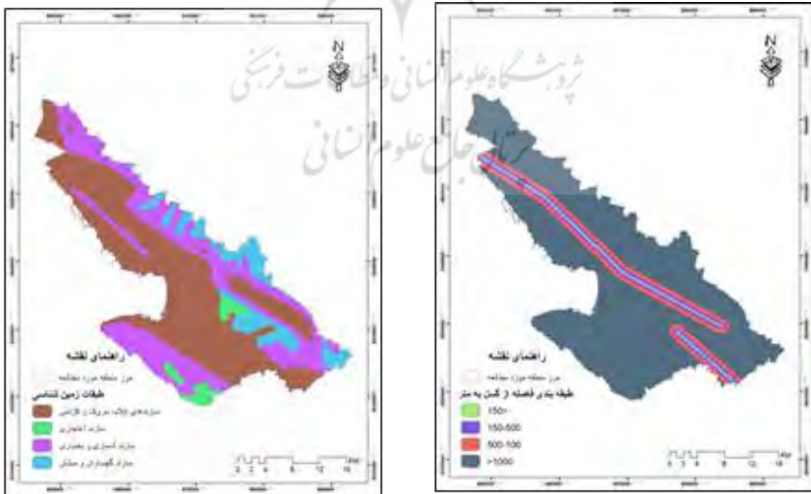
شکل ۱۲- طبقه بندی فاصله از گسل شکل ۱۳- طبقات زمین شناسی محدوده مورد مطالعه
