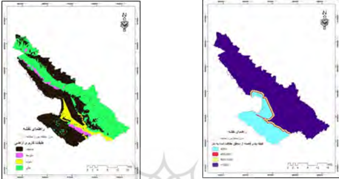
شکل ۱۰- طبقه بندی فاصله از مناطق حفاظت شده - شکل ۱۱- طبقه بندی کاربری اراضی محدوده مورد مطالعه
