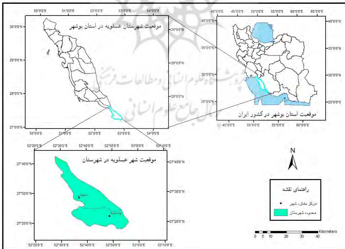
شکل ۱- موقعیت جغرافیایی محدوده مورد مطالعه Source: Research findings
