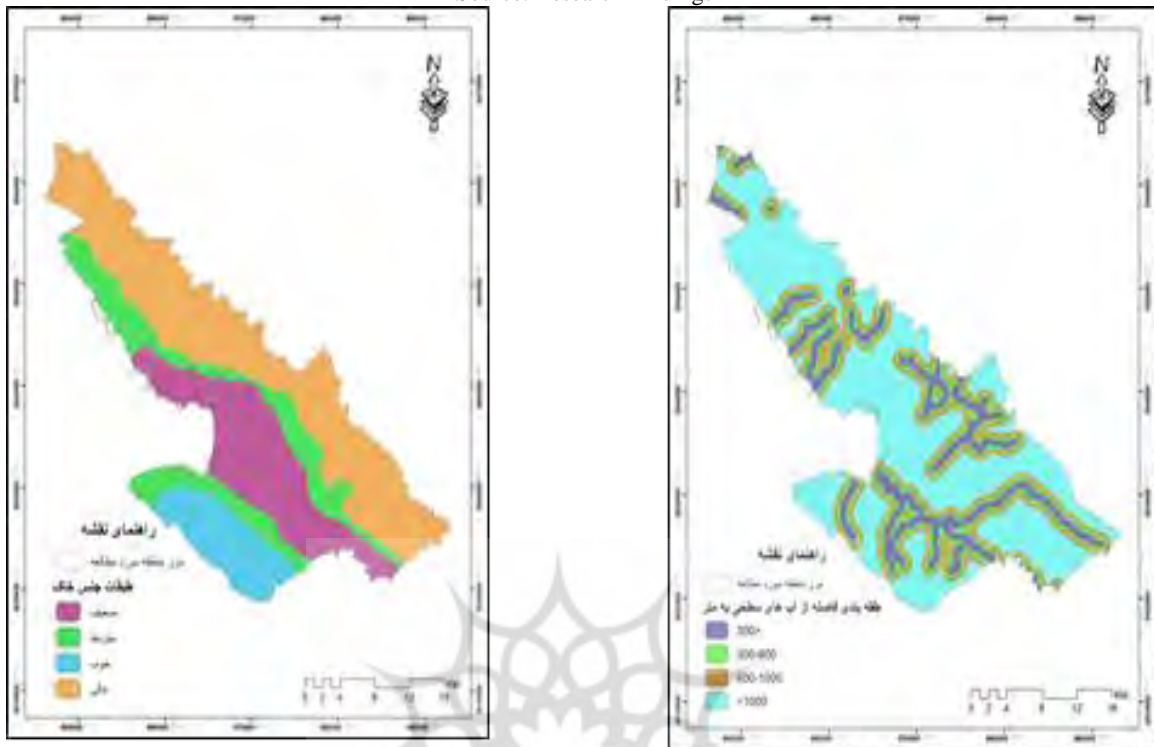
شکل ۱۴- طبقات خاک محدوده مورد مطالعه شکل ۱۵- طبقه بندی فاصله از آب‌های سطحی
