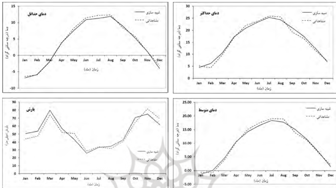
شکل ۲: مقایسه مقادیر دما و بارش ماهانه داده‌های مشاهده شده و شبیه‌سازی شده در مرحله اعتبارسنجی مدل
