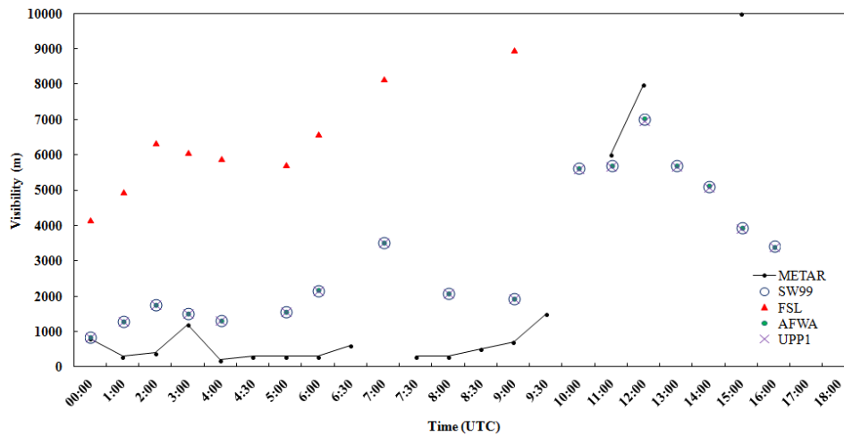
شکل ۳: مانند شکل ۲ ولی در فرودگاه مهرآباد تهران.
