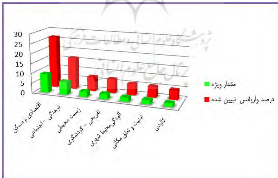
شکل (۲): مقدار ویژه و درصد واریانس تبیین شده عوامل مهاجرت معکوس
