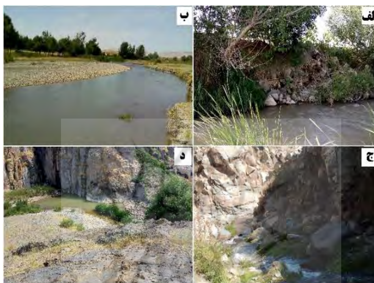
شکل ۱۰- الف و ب: فرسایش کنار رودخانه به علت وجود مواد سست و فرسایش پذیر؛ ج و د: مقاومت زمین‌شناسی کنار رودخانه و عرض کم منتج از این عامل
