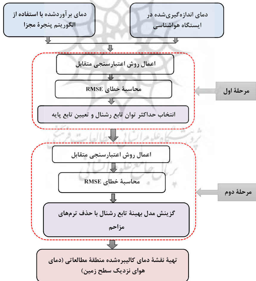
شکل ۴. فلوچارت روش کالیبراسیون مورد استفاده در پژوهش حاضر، به منظور برآورد دمای هوای نزدیک سطح زمین
