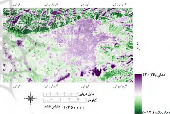
نگاره ۳: دمای سطح زمین استخراجی از تصویر سنجنده TIR در تاریخ ۱۶-آذر-۱۳۹۶
