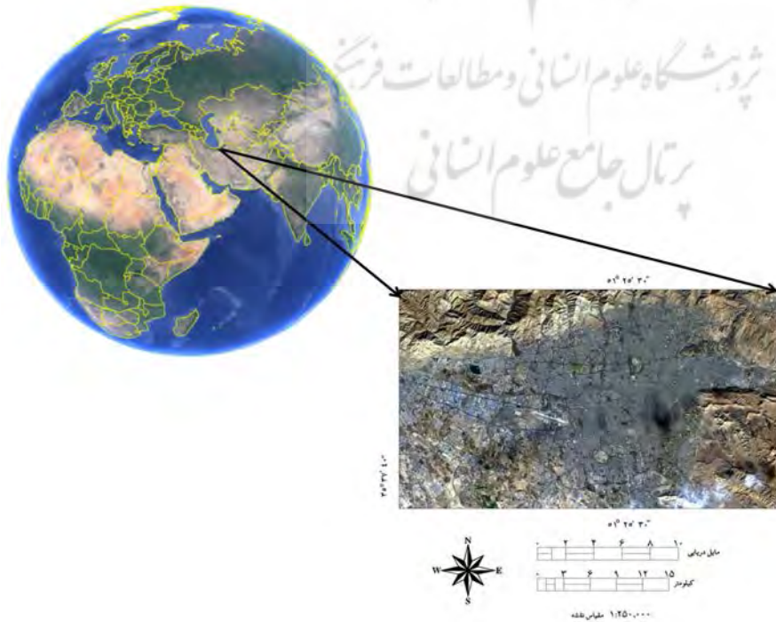
نگاره ۱: موقعیت منطقه مطالعاتی؛ تصویر ماهواره سال ۲۰۱۸ میلادی از تهران که از ترکیب باندهای (۲) = ۴۸۲/۰ میکرومتر، (باندها ۳) = ۵۶۱/۰ میکرومتر و باندها (۴) = ۶۵۴/۰ میکرومتر است
