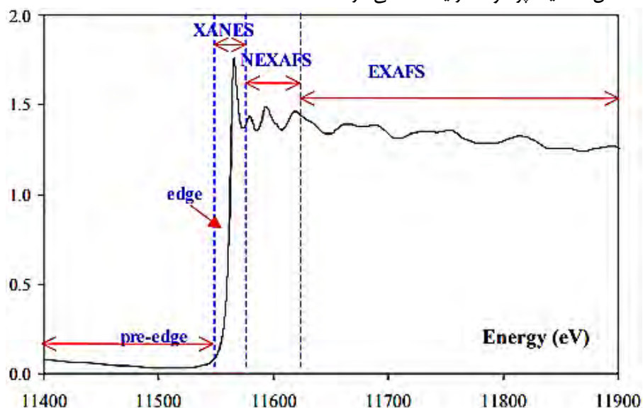
شکل ۷: نواحی مختلف طیف جذبی پرتویکس [14]
