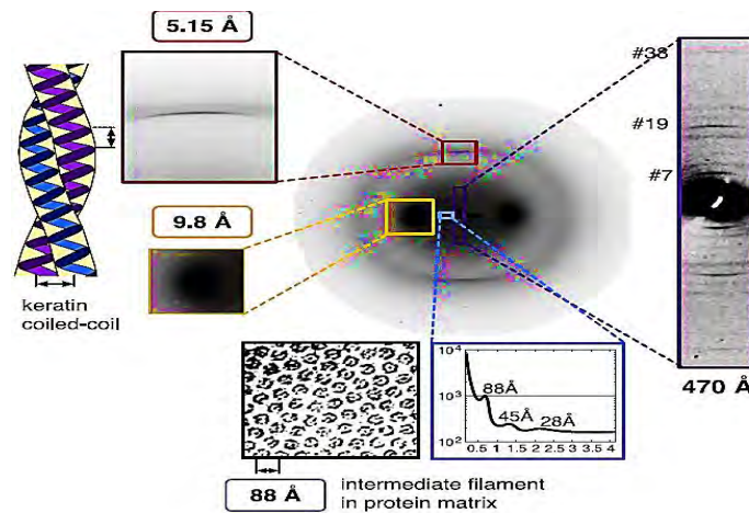
شکل ۱۰: تصویر SAXS از موی یک مومیایی مصر باستان، ابر مولکول‌های موجود در کراتین -آلفا با قابلیت وضوح آنگستروم از ماکرو مولکول‌های موجود در آن تشخیص پذیر هستند [26].
