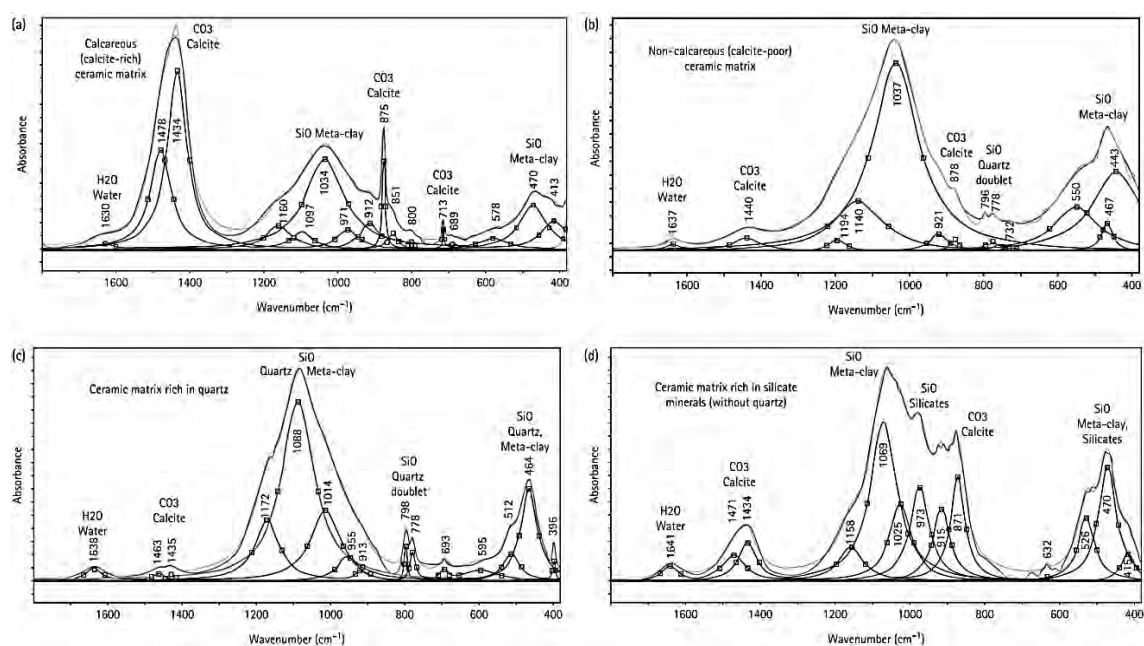
شکل ۱۱: داده‌های برازش شده طیف‌های FT-IR مواد سرامیکی از سفال‌های سرامیک سرپاچه‌های لوانتین [28]
