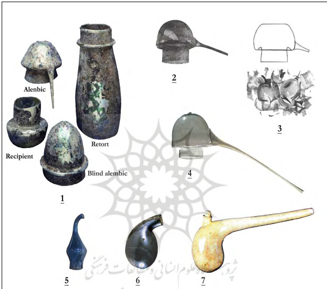
شکل ۱: ظروف تقطیر دوران اسلامی تا معاصر
