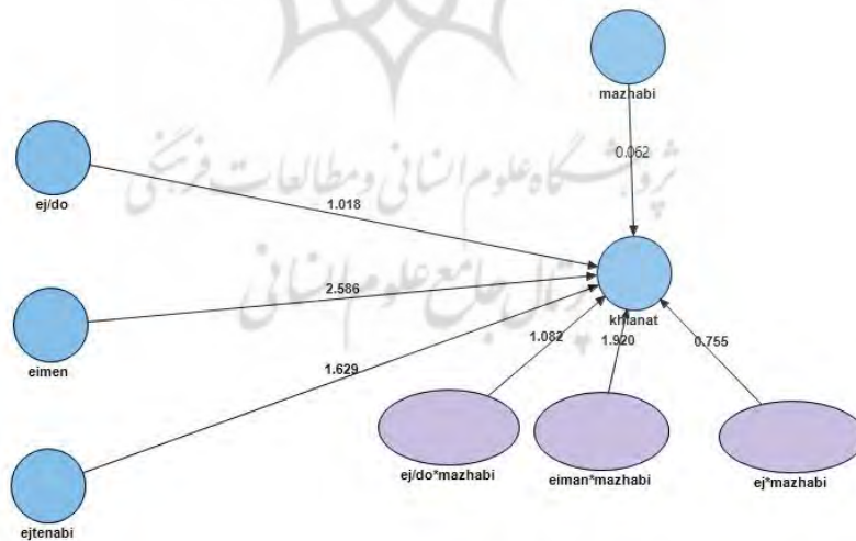
نمودار ۴. مدل تحلیل مسیر پس از محاسبه ضرایب t مسیر میان متغیرها با تعدیل‌گر
