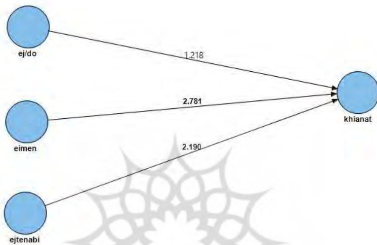
نمودار ۳. مدل تحلیل مسیر پس از محاسبه t مسیر میان متغیرها بدون تعدیل‌گر
