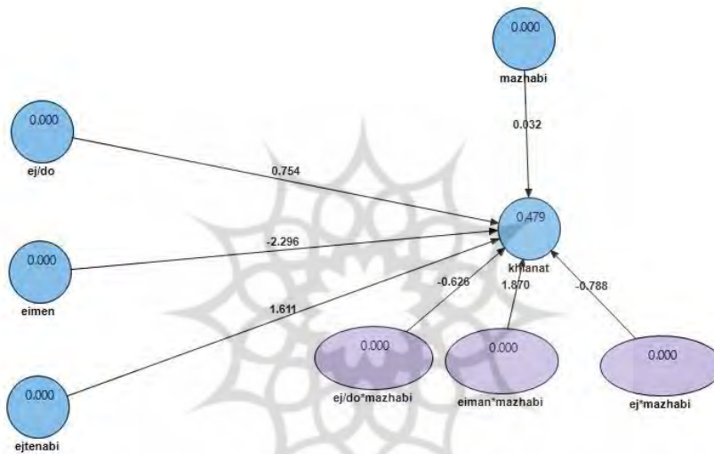
نمودار ۲. مدل تحلیل مسیر پس از محاسبه ضرایب مسیر میان متغیرها با تعدیل‌گر
