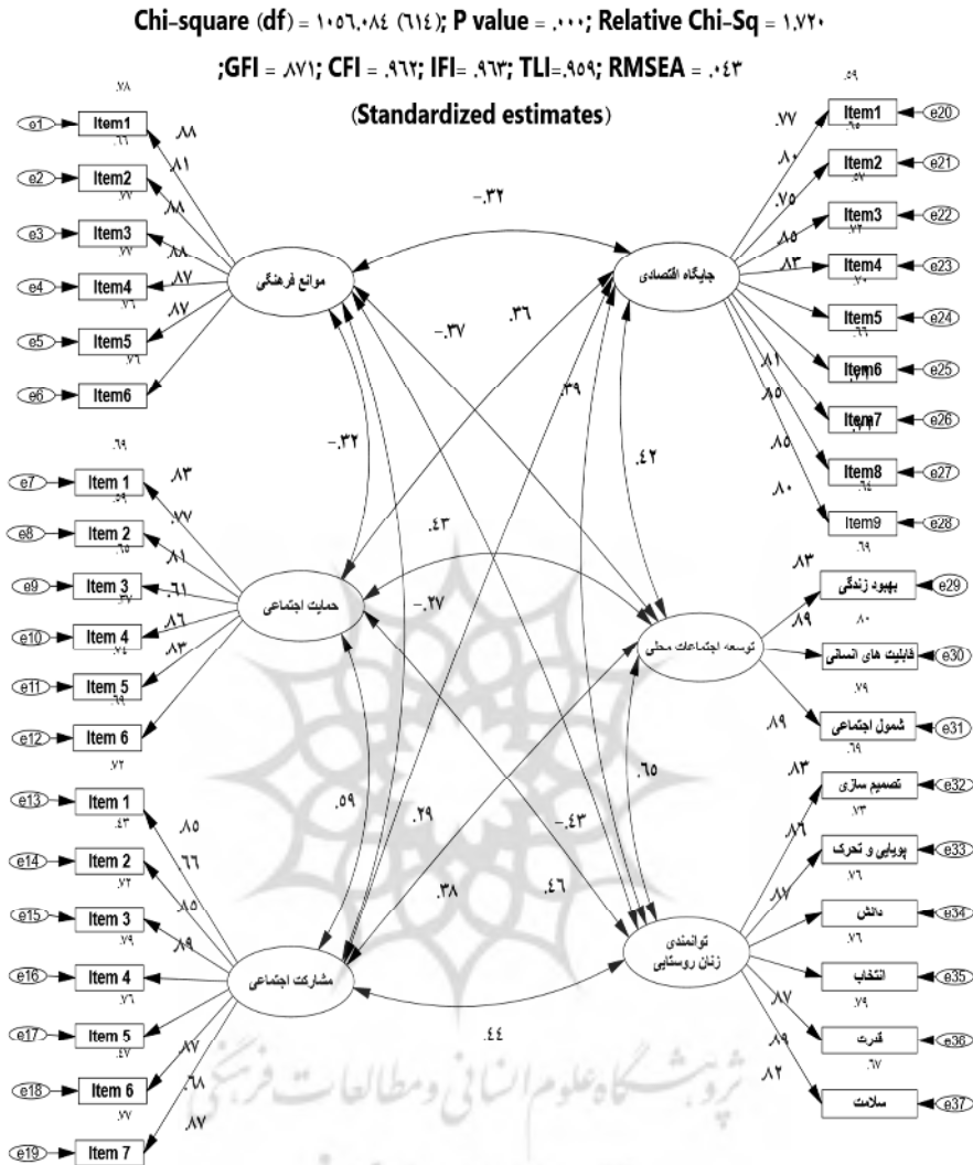
شکل ۲- مدل اندازه گیری بر اساس مقادیر عاملی استاندارد
