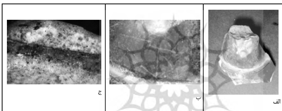
تصویر ۳: الف. نمونه M111 ب. تصویر میکروسکوپی با بزرگنمایی X250، بخش‌های برجسته، زرانود و قلم‌گیری را نشان می‌دهد. ج. تصویر میکروسکوپی از سطح مقطع، قرارگیری لایه طلا را در سطح لعاب و محصور شدن لعاب زمینه بین بدنه و بخش برجسته را به‌وضوح نشان می‌دهد.
