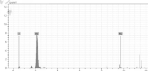
نمودار ۱: EDX بخش زراندود در سفال مینایی M111 حضور طلای خالص را نشان می‌دهد.
