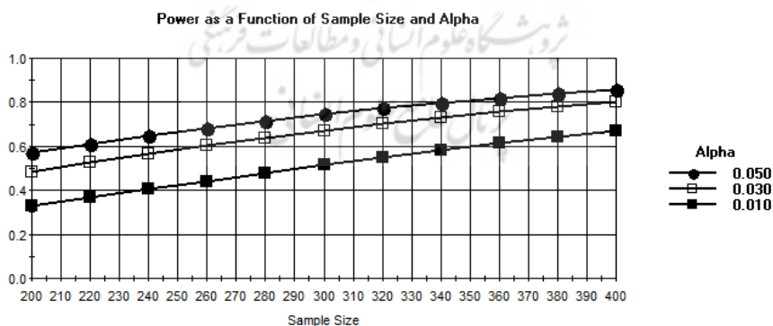
نمودار ۱: برآورد حجم نمونه بر اساس تحلیل توان در سطح آلفای‌های مختلف
