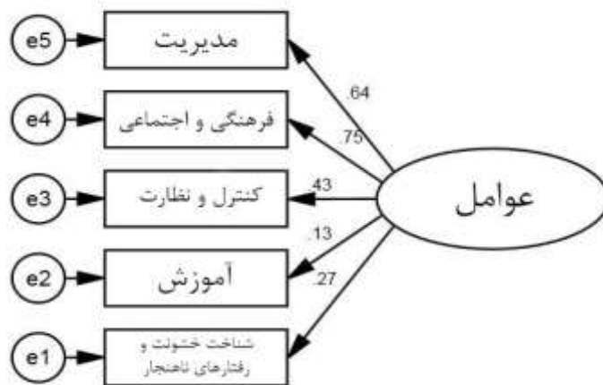
شکل ۲- تحلیل عاملی تأییدی مرتبه‌ی دوم
