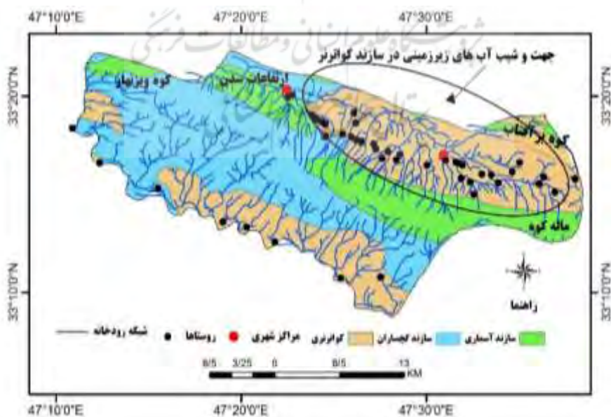
شکل ۴. شیب آب‌های زیرزمینی منطقه رومشکان در سازند کواترن
