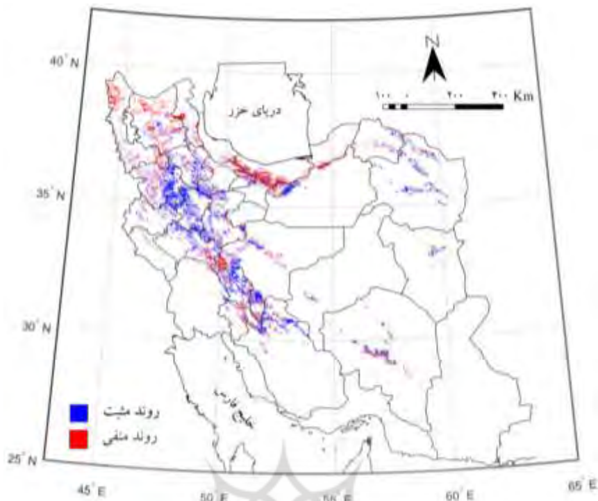
شکل ۴. روند تغییرات مکانی آغاز فصل انباشت پوشش برف در ایران بدون در نظر گرفتن میزان تغییرات
