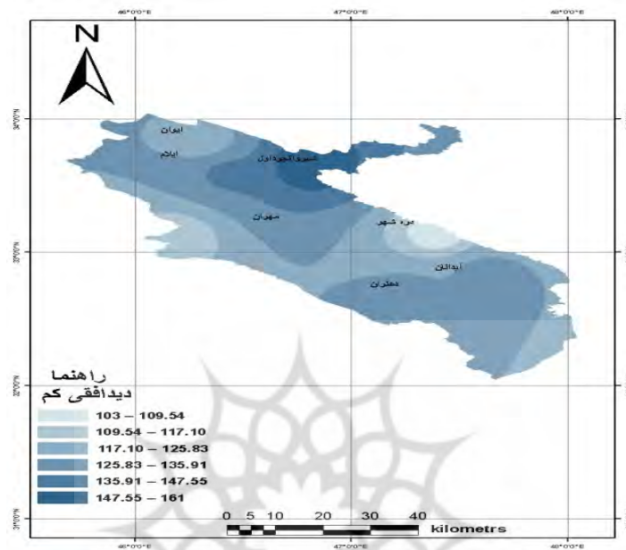
شکل (۸) تعداد روزهای با دید کم برحسب (دید افقی کمتر از ۱۰ کیلومتر) در استان ایلام
