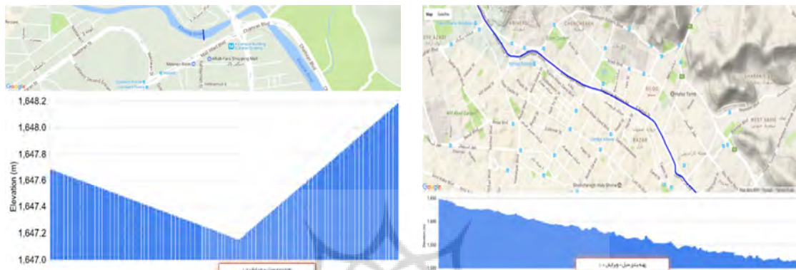
شکل ۲: پروفیل طولی (شکل سمت راست) و پروفیل عرضی (شکل سمت چپ) رودخانه خشک شیراز-فارس
