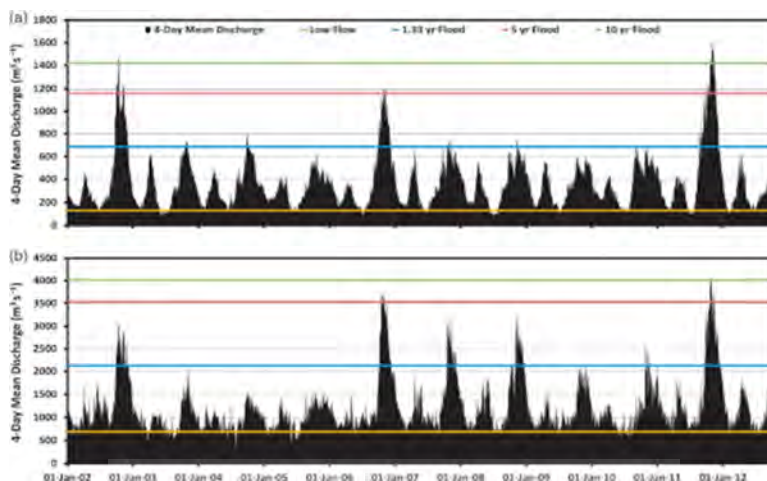
شکل ۱۲: هیدروگراف سیل ۲۳ اکتبر ۲۰۱۱ شهر آبوتایا-تایلند (شکل a و b هیدروگراف قبل و پس از اتصال دو شاخه رودخانه است).
