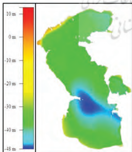
نگاره ۵: تغییرات جهانی MSS در دریای خزر
