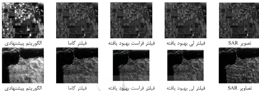
شکل ۱۱. خروجی فیلترهای مختلف بر روی تصاویر SAR هوایی، به ترتیب از بالا به پایین تصویر فلولاند و تصویر سانفرانسیسکو (تصاویر "الف" و "ب")
