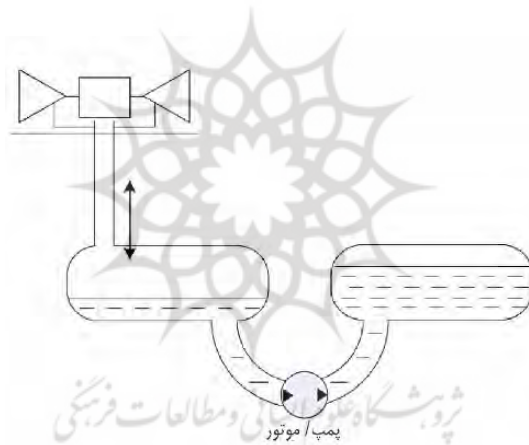
شکل ۵. نمای شماتیک سیستم ترکیبی ذخیره‌سازی انرژی هوای فشرده-تلمبه‌ذخیره‌ای فشارثابت [۳۱]
