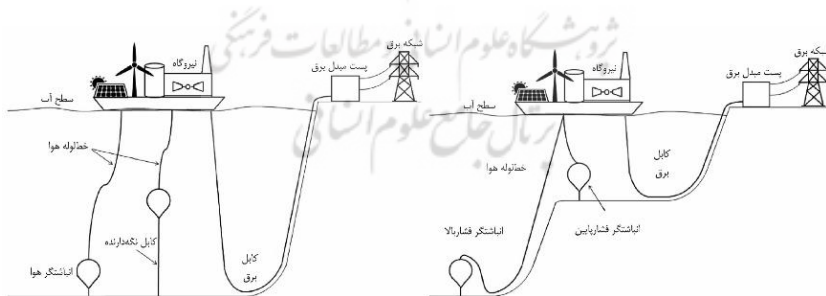
شکل ۹. نمونه‌هایی از طراحی‌های پیشنهادی برای سیستم ذخیره‌سازی انرژی هوای فشرده زیرآبی چندسطحی [۵۵]
