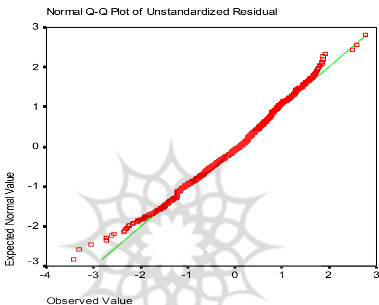
نمودار ۲- بررسی نرمالیتی خطاهای مدل
