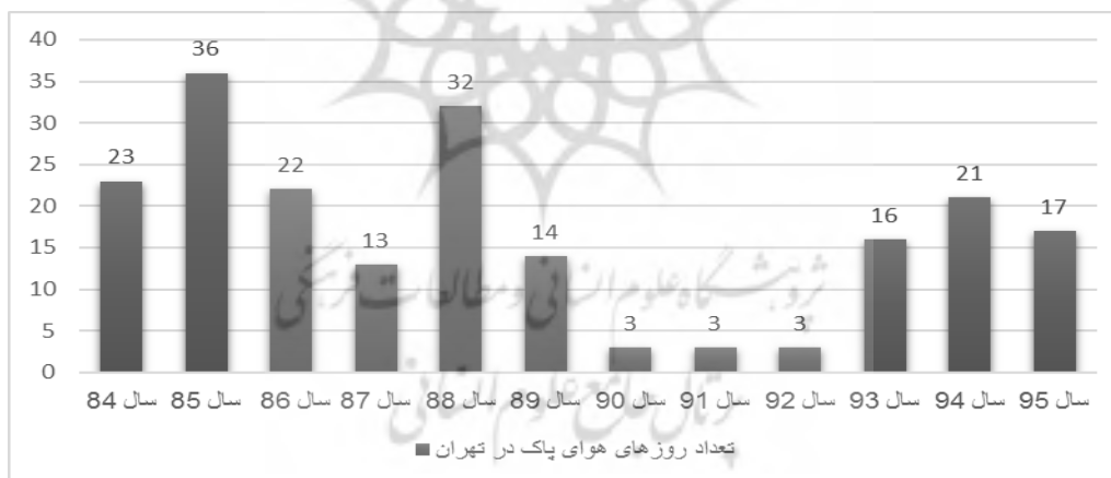
نمودار ۱۰: تعداد روزهای پاک در سطح شهر تهران در سال‌های ۹۵-۸۴ http://tmicto.tehran.ir&author;2019 Source:
