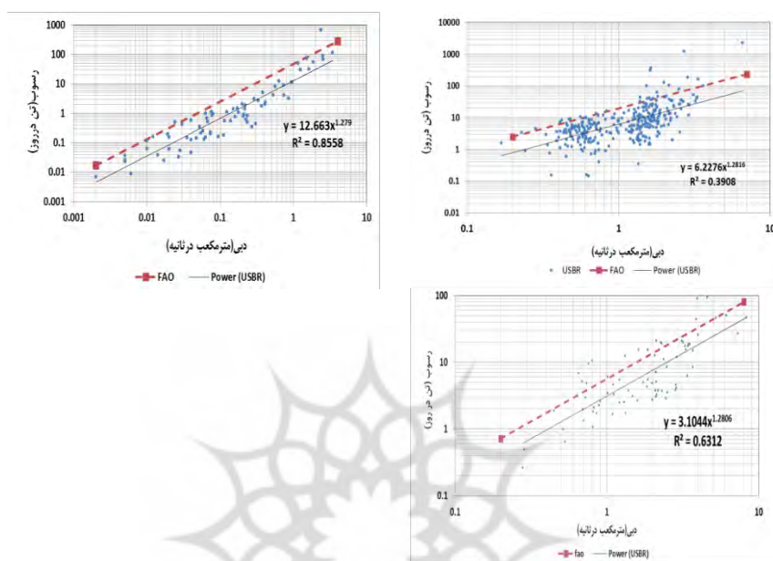
شکل ۵- نمودار همبستگی نمایی دبی و رسوب رودخانه در حوضه‌های الف) آتشگاه، ب) عموقین، پ) کوزه توپراقی، ت) نوران، ث) نیر، ج) باروق و چ) یامچی
