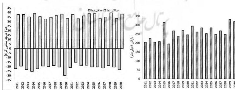
شکل ۲- نتایج پیش‌بینی مدل Lars با سناریو A1B: الف) بارندگی، ب) درجه حرارت حداقل و حداکثر
