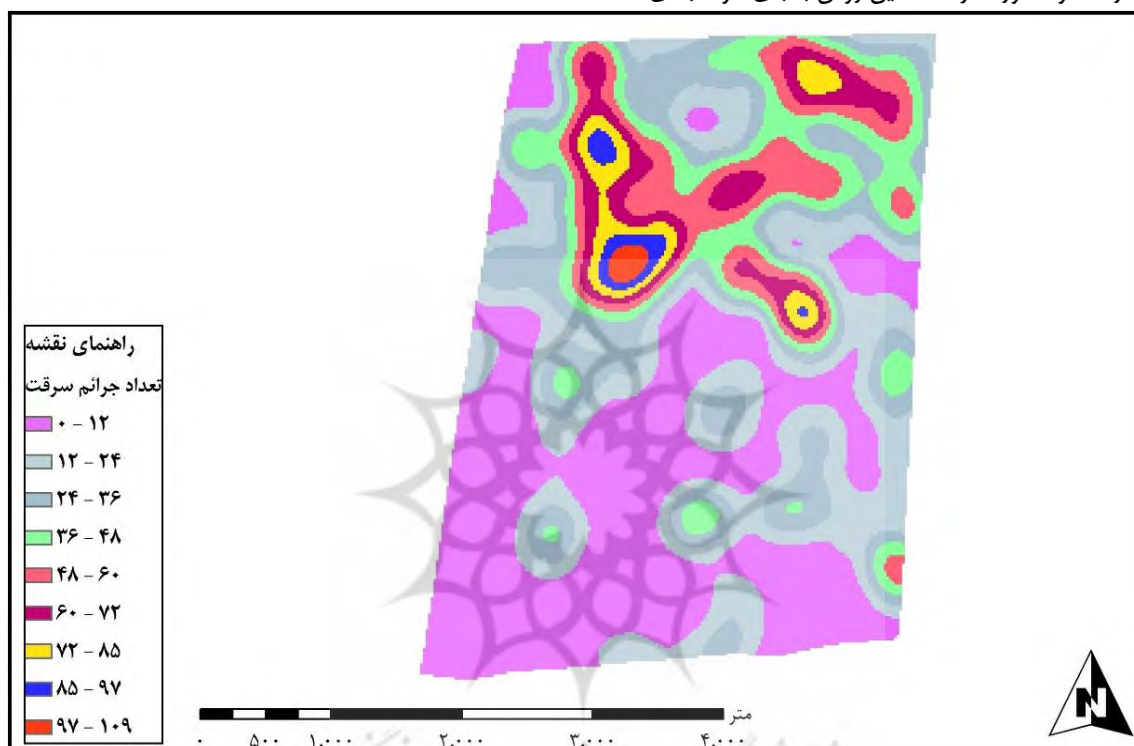
شکل ۲. تراکم کرنل جرائم سرقت محدوده مورد مطالعه
