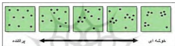
شکل ۴. نمایش شماتیک خوشه‌ای یا پراکنده بودن داده‌های فضایی
