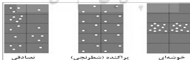
شکل ۳. الگوهای خوشه‌ای، پراکنده و تصادفی گسترش فیزیکی شهر
