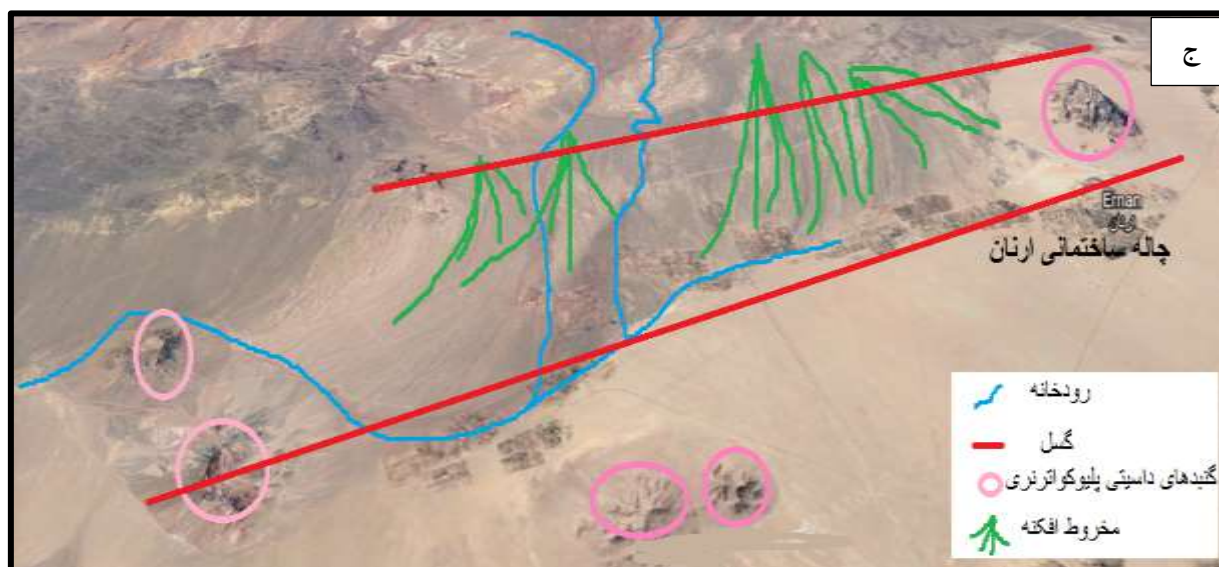
شکل ۳. الف. بریده‌شدن مخروط‌افکنه‌ها و رسوبات جدید بر اثر گسل دهشیر در تصویر ماهواره‌ای؛ ب. اثر گسل دهشیر و بالآآمدگی رسوبات عهد حاضر (دید به سوی شمال خاور)؛ پ. بریده‌شدن رسوبات رودخانه‌ای؛ ت. اثر گسل دهشیر بر واحدهای افیولیتی (دید به سوی جنوب)؛ ج. بریده‌شدن رأس مخروط‌افکنه‌ها و تغییر در الگوی شبکه زهکشی بر اثر فعالیت گسل‌ها در پیرامون چاله ارنان در کوآترنری (منبع: نویسندگان، ۱۳۹۸).
