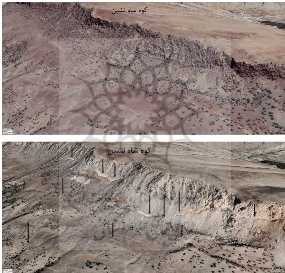
شکل (۳). زبانه های لغزشی در پای کوه شاه نشین ناشی از وقوع زمین لرزه ازگله.
